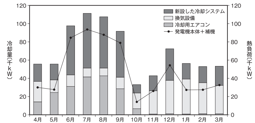
図3 熱負荷と冷却量の推移
