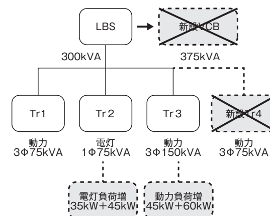
図2 最終解決案の幹線系統図
